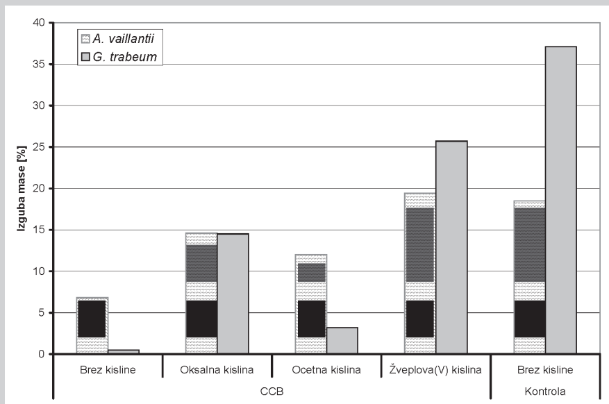
Slika 1. Izgube mase kontrolnih in s CCB impregniranih vzorcev, prepojenih z različnimi kislinami po osmih tednih delovanja na baker tolerantne bele hišne gobe ( A. vaillantii ) in na baker občutljive tramovke ( G. trabeum ) (Humar et al., 2005)
