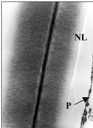
Slika 4: Oktober 2001 - nediferencirane celične stene terminalnih traheid kasnega lesa ob kambiju pri jelkah s širšimi branikami. Sekundarna celična stena ni dokončno oblikovana, notranji sloji so nelignificirani (NL). V lumnu so vidni ostanki protoplazme (P). Povečava:9300x
