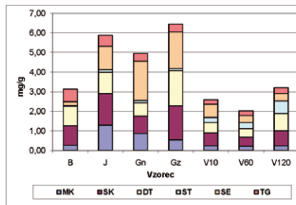
Slika 2. Sestava lipofilne frakcije v lesnih tkivih na višini 13 m (B-beljava, J-jedrovina, Gn, Gz-notranja in zunanja polovica grče, V10, V60, V120-segmenti veje)
